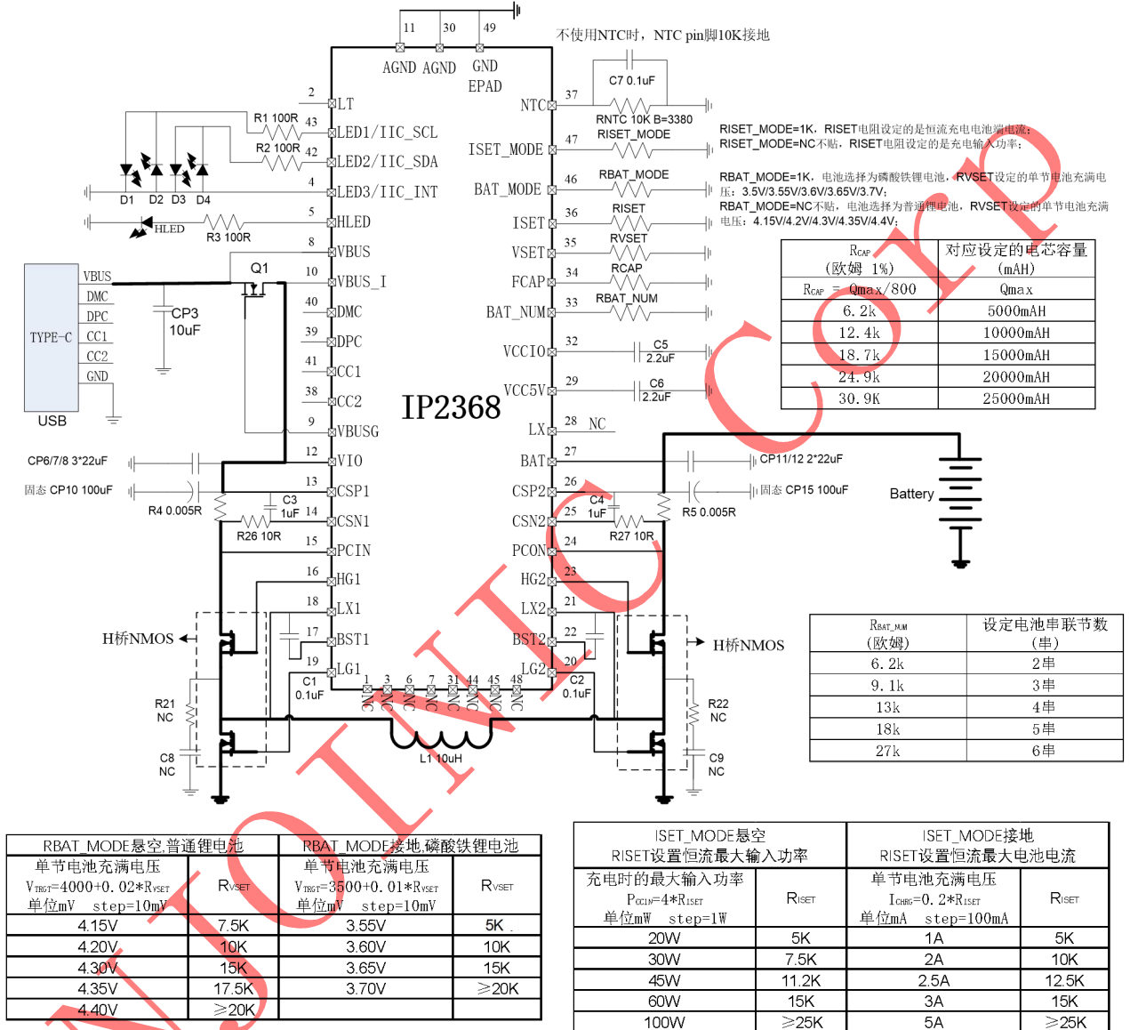
图 13 应用原理图
