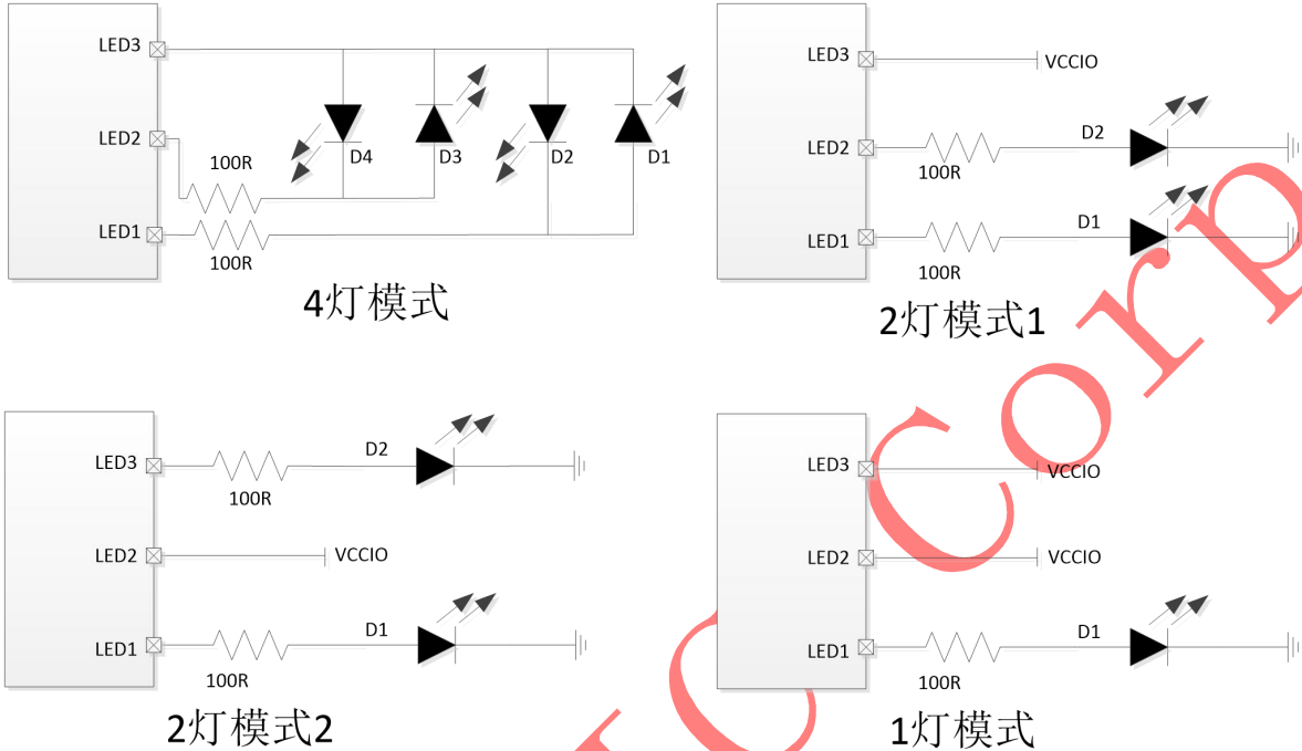
4、2、1 LED 连接方式
